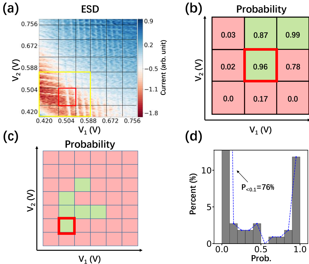
图 3.9 少电子区的搜索过程。(a) 双量子点的电荷稳定图。在处理过程中相图按照约 0.06 \text{ V} \times 0.06 \text{ V} (31 px) 的大小被划分为多个部分,在此例中相图被分为 42 个部分,每一个部分将分别由 CNN 进行识别并分类。(b) CNN 给出的电荷稳定图中各区域处于双点状态的概率。图中给出了一部分详细的概率值,概率值高于 80% 的部分被记录为双点态,低于 80% 的部分被记录为非双点态,分别使用绿色和红色标注。(c) 完整电荷稳定图中由 CNN 给出的各区域处于双点态的概率。少电子区通过选取概率高于 80% 的区域中拥有最低电压的部分进行定位。结果由红色框标注。(d) 相图中电荷态识别的概率分布直方图。
